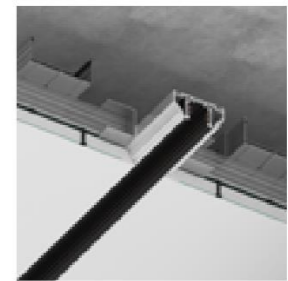
Монтаж в один слой гипсокартона
