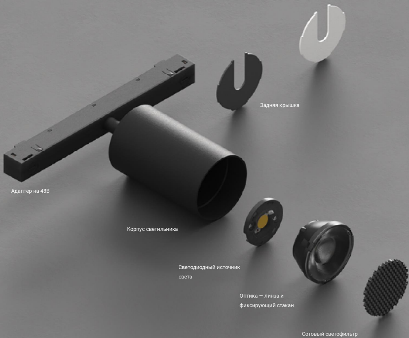
Сотовый светофильтр
